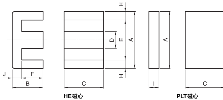
HE磁心
