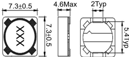
unit:mm
