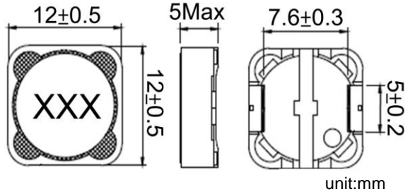
unit:mm
