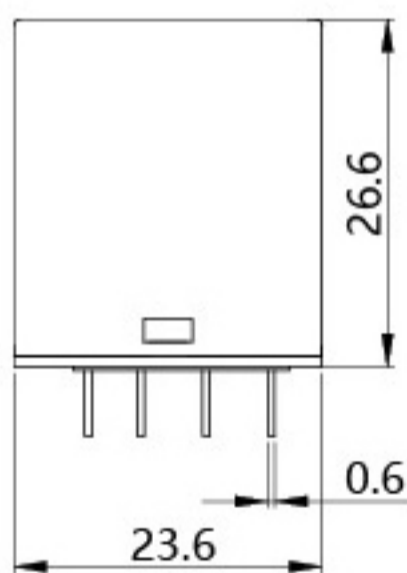
正面图
