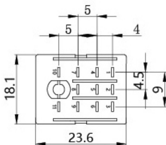
安装尺寸
