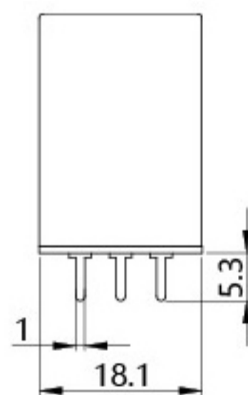
侧面图
