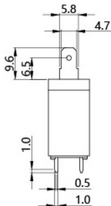
侧面图
