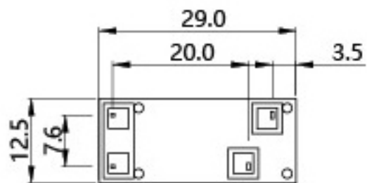
安装尺寸
