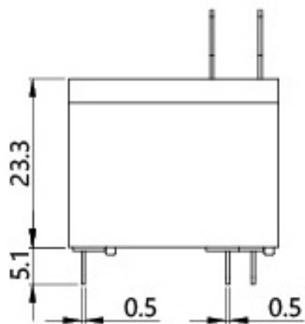
正面图
