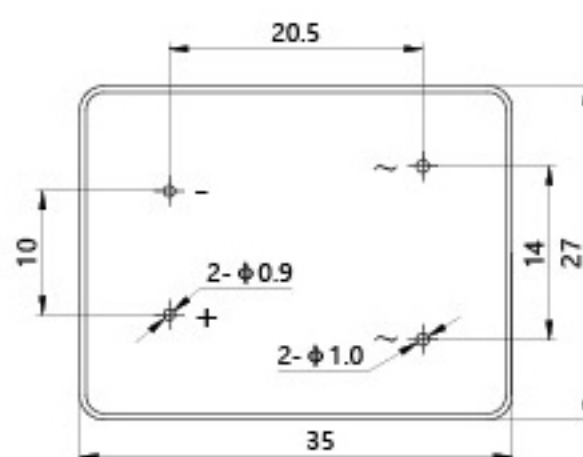
安装尺寸
