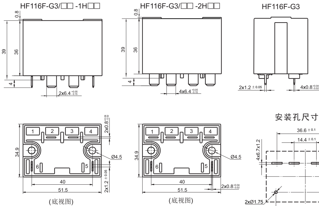
外形图
