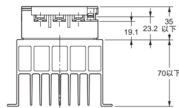
端子配置/内部连接
