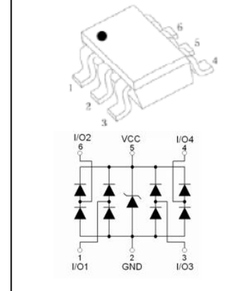
SOT-23-6L
