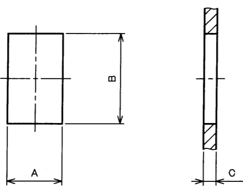
パネル取付寸法
